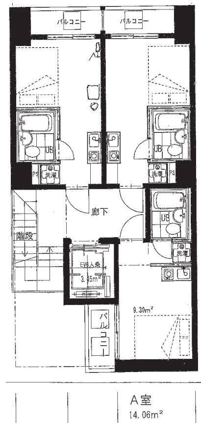
1階平面図 S=1/100 2～6階平面図 S=1/100
