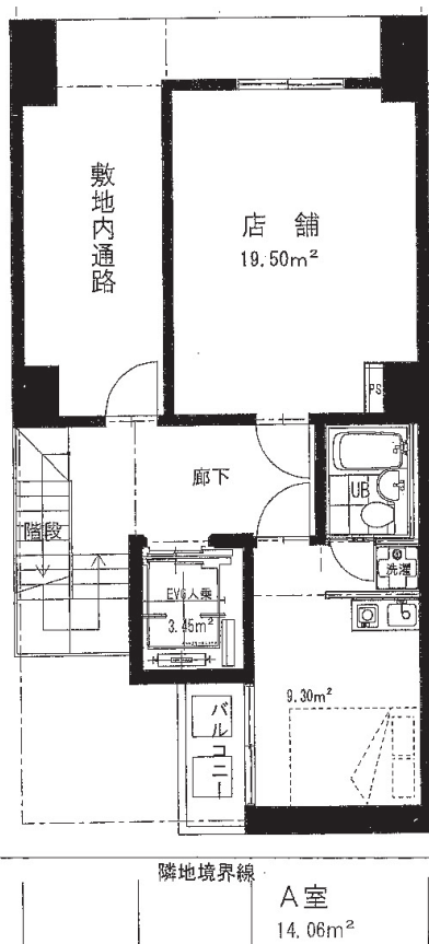
1階平面図 S=1/100 2～6階平面図 S=1/100
